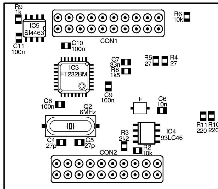
Rysunek 4: Rozmieszczenie elementów na płytce, widok z dołu.
