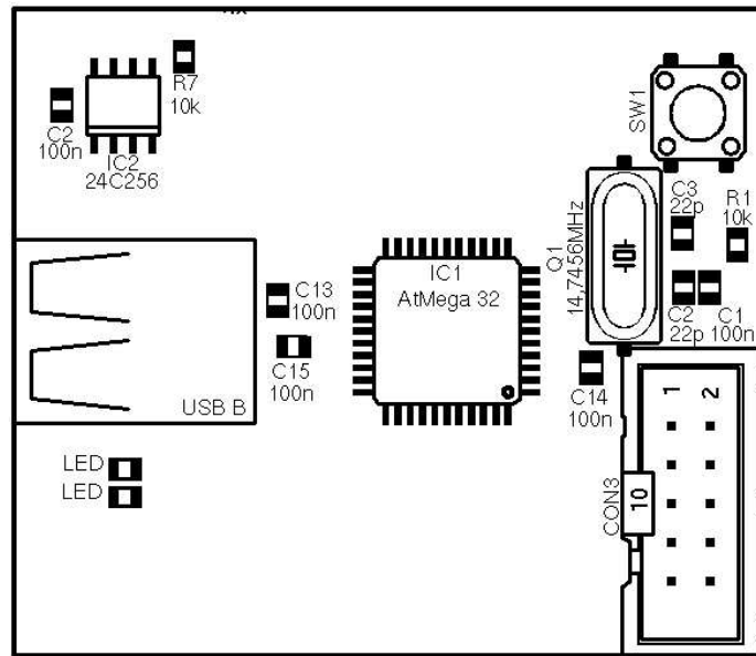
Rysunek 3: Rozmieszczenie elementów na płytce, widok z góry.
